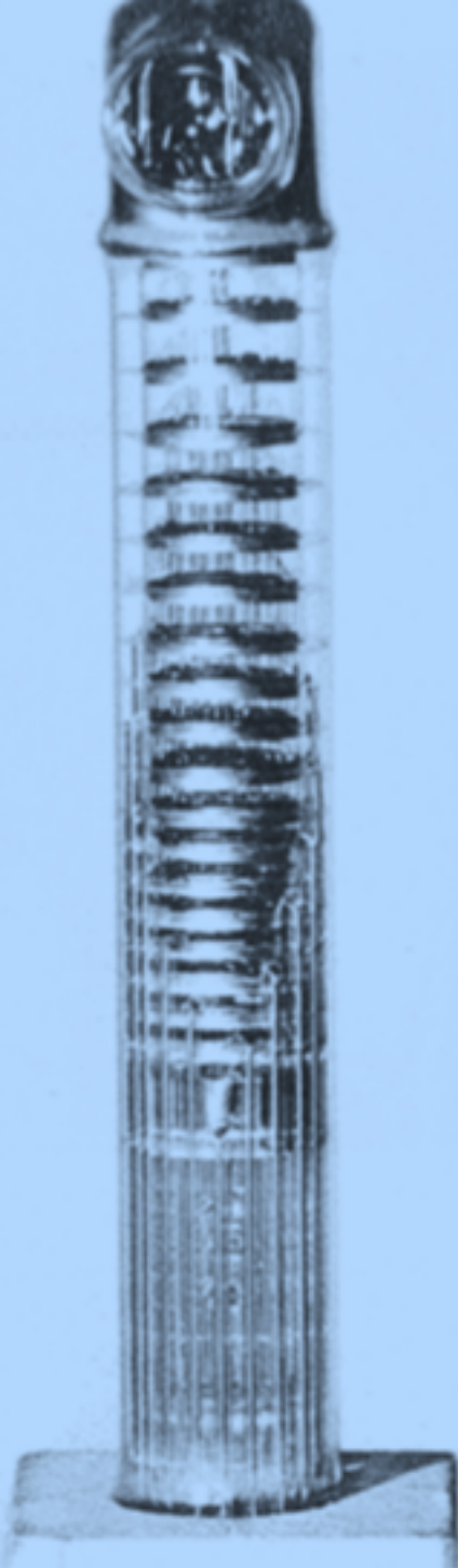
Photo-multiplificateur de l'Observatoire de Paris, sensible à la lumière ultra-violette, à 20 étages, dimensions: 38 cm.-6cm.
